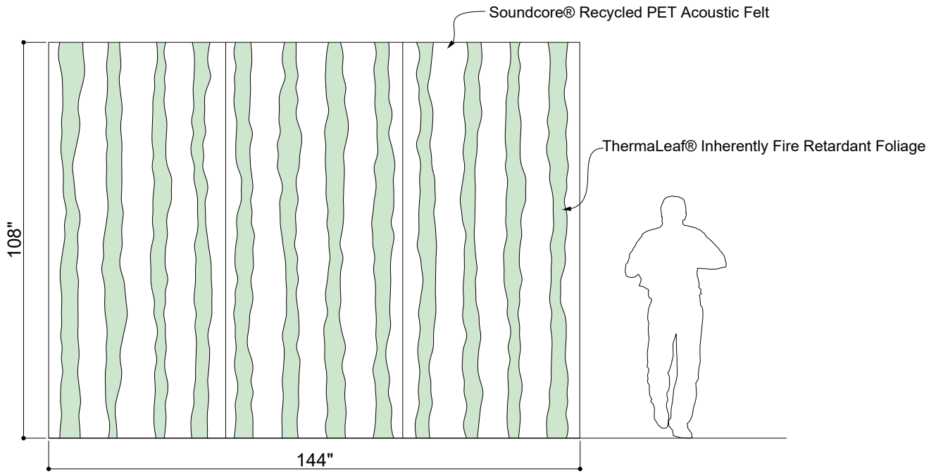
① ELEVATION 2
