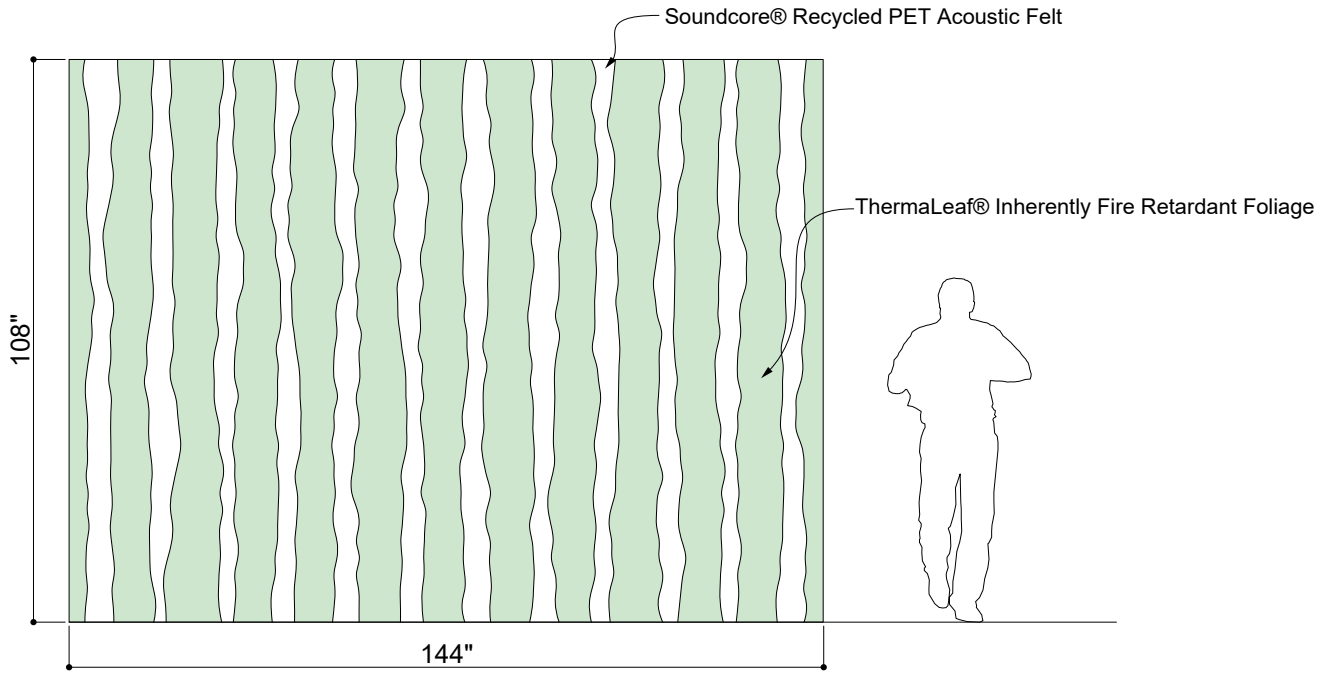
① ELEVATION 1
